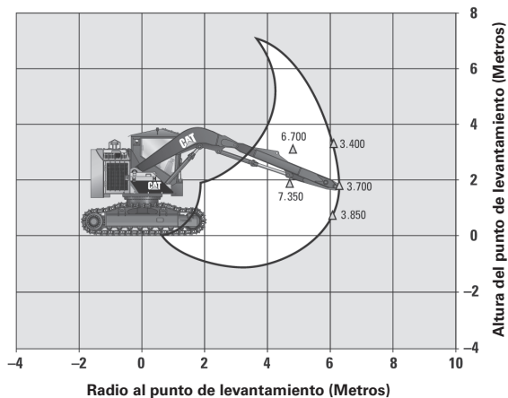
Información de alcance de levantamiento: Barrido de pluma de culata fija 501HD
