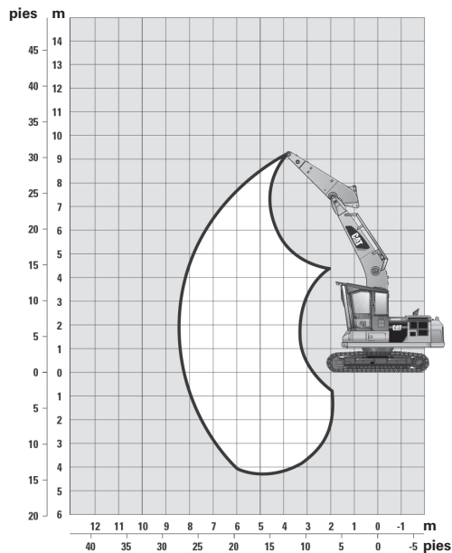
Forestal general Brazo de 2,9 m (9' 6")
