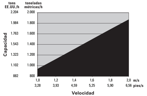
Rendimiento de transporte del cárter de línea del sistema AFC: PF4/832
