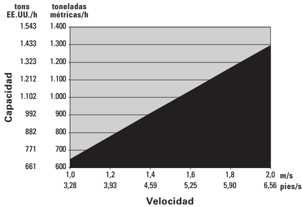
Rendimiento de transporte del cárter de línea del sistema AFC: PF3/722
