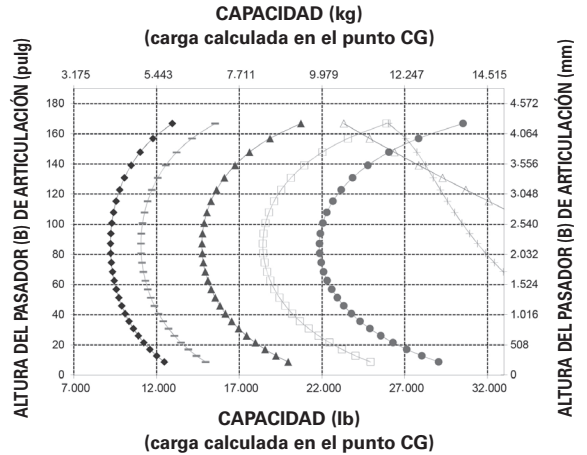
962M LOG Horquilla de garfio UFO, Comp QC Volvo
