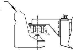
Adaptador de enganche de la 5ª rueda del CL215
