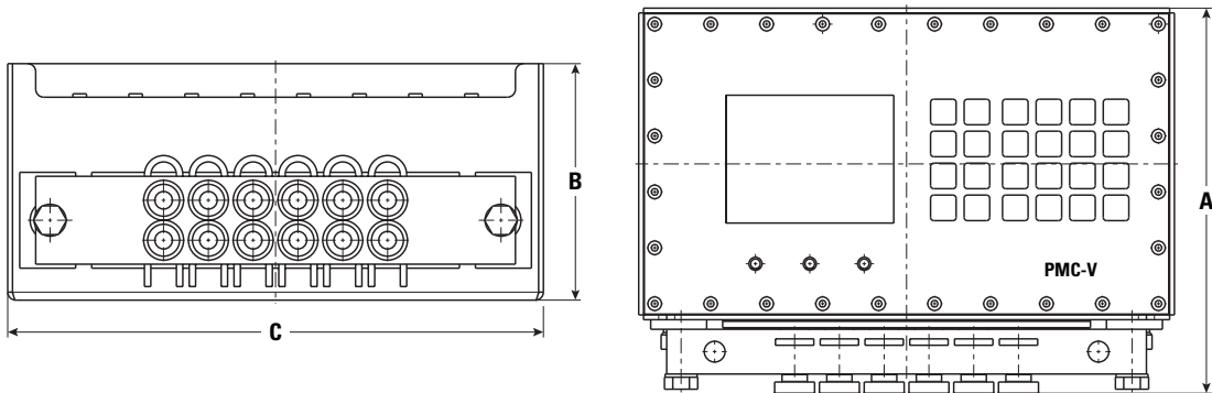
Dimensiones de PMC-V (todas las dimensiones son aproximadas).
