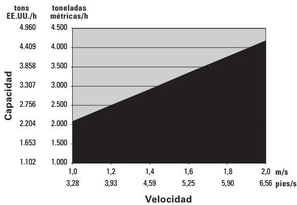
Rendimiento de transporte del cárter de línea del sistema AFC: PF4
