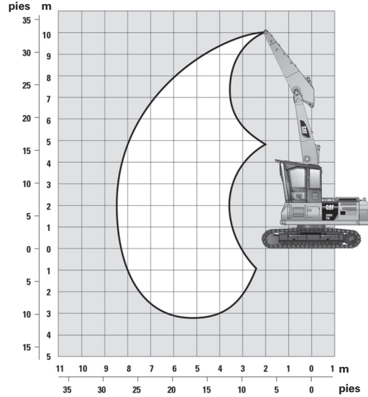
Cargador de troncos HD/LC Pluma recta de 5,7 m (18' 8") con brazo R2.9B1 (9' 6")
