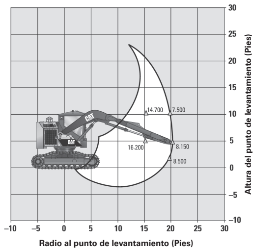
Información de alcance de levantamiento: Barrido de pluma de culata fija 501HD
