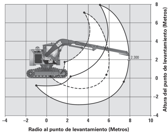
Información de alcance de levantamiento: Barrido de pluma telescópica 501HD
