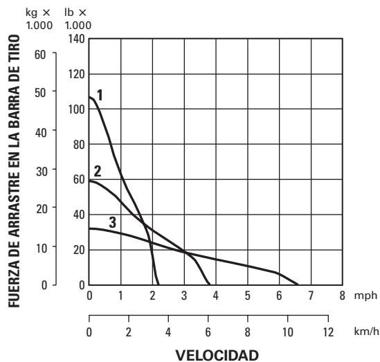
Dirección diferencial de D7R estándar/XR/LGP
