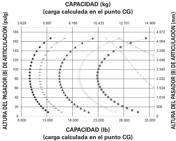
962M LOG Horquilla de garfio UFO, Fusion
