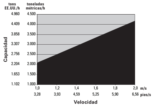
Rendimiento de transporte del cárter de línea del sistema AFC: PF5
