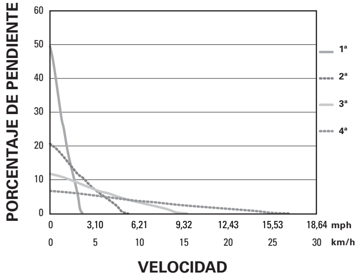
CL215 % DE PENDIENTE frente a VELOCIDAD: CARGADO
