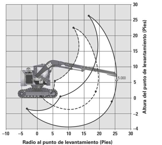
Información de alcance de levantamiento: Barrido de pluma telescópica 501HD
