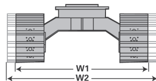
Cosechadoras de cadena 522B (inclinable) ZTS
