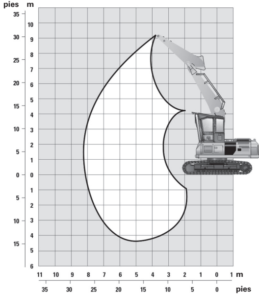
Cargador de troncos HD/LC Pluma curva HD R de 5,7 m (18' 8") con brazo R2.9B1 (9' 6")
