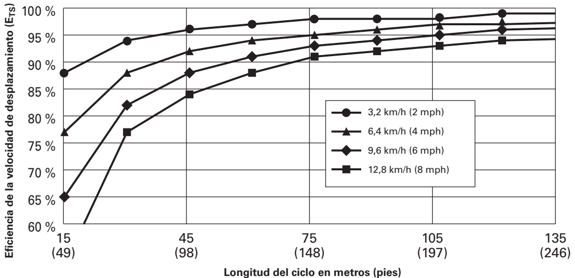
Eficiencia de la velocidad de desplazamiento
