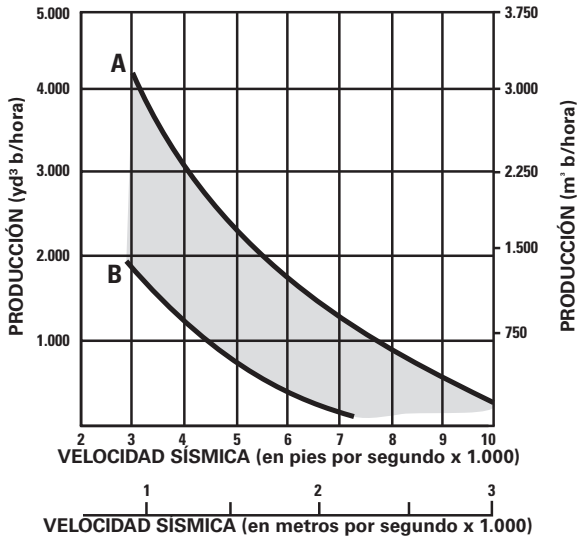
D11T CD CON VÁSTAGO SENCILLO
